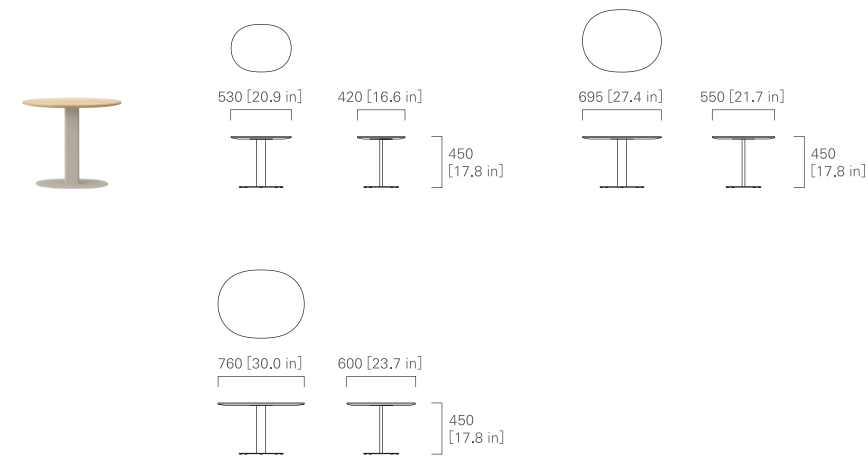
LOBBY TABLE 53, 70, 76 (oval)
