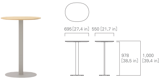
BAR TABLE 70 High (oval)
