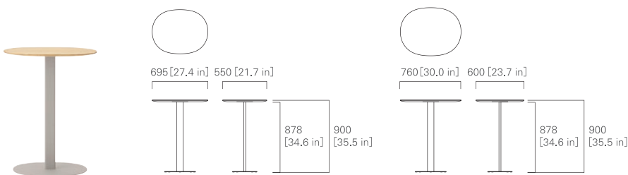
BAR TABLE 70, 76 Mid (oval)
