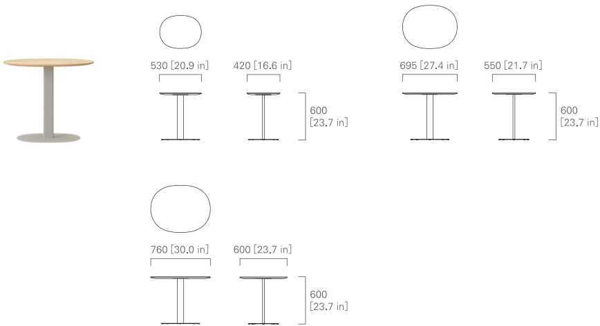
LOBBY TABLE 53, 70, 76 (oval)
