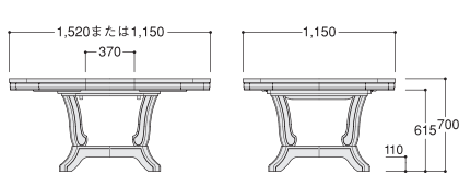
No.1409-00 パーティテーブル (シンクロスライド)
