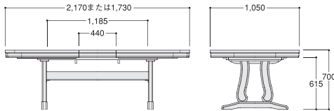
No.1410-00 ダイニングテーブル (シンクロスライド)
