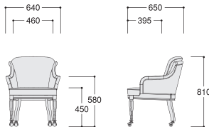
No.2409-01 パーティチェア
