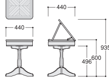
No.3410-00 サイドテーブル
