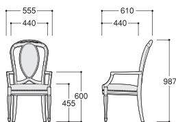
No.2410-01 チェア(肘付)
