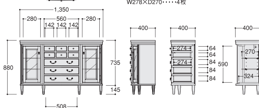
No.6573-01 サイドボード135
