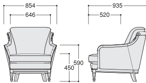
No.4410-01 アームチェア
