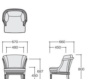
No.2698-11 パーティチェア (キャスター無し)
