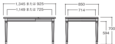
No.1795-10 ダイニングテーブル (片バタ式)
