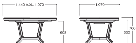
No.1809-00 パーティテーブル (シンクロスライド)
