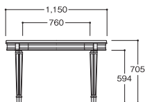
No.1777-00 パーティテーブル115
